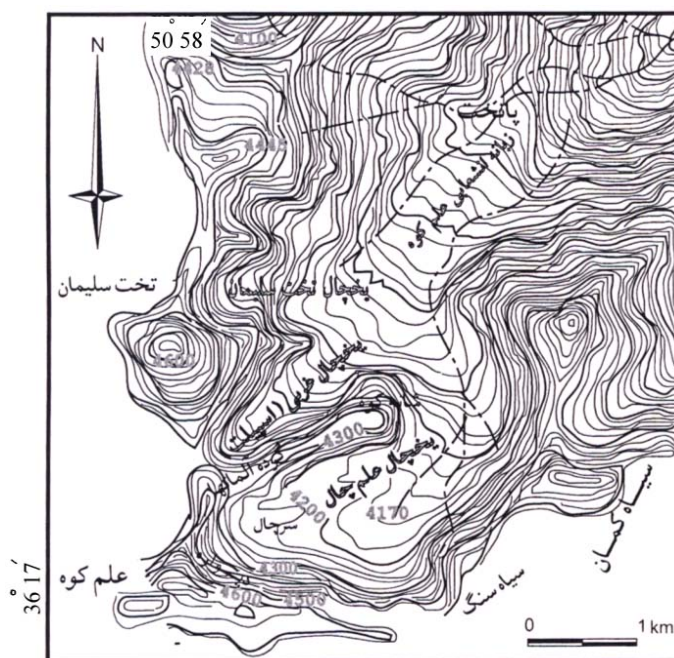
شکل ۱. توپوگرافی محدوده یخچال‌های علم‌کوه
