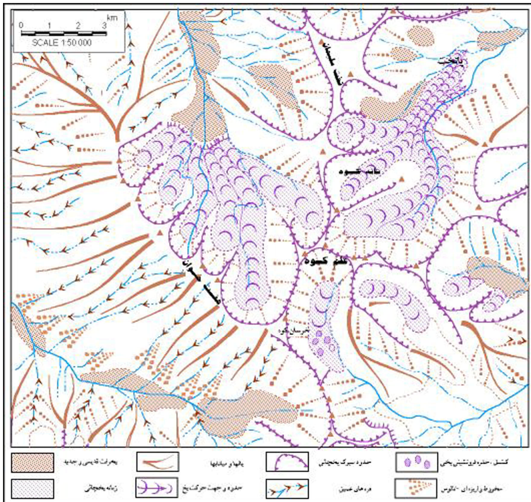
شکل ۱۲. زبانه‌های یخچالی مورد مطالعه در دامنه شمالی علم‌کوه
