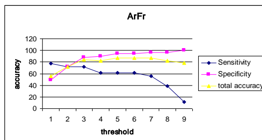
شکل ۱۳. نمودار حساسیت، خصوصیت و صحت کلی در احتمالات مختلف
