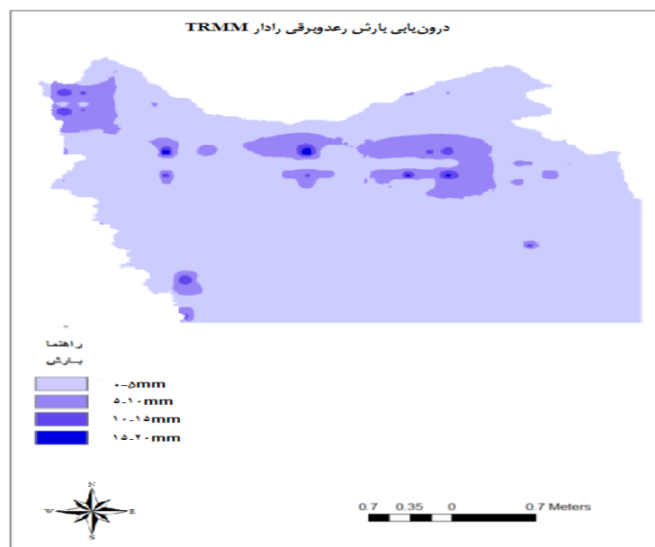
شکل ۴. تصویر درون‌یابی بارش رعدوبرقی رادار TRMM روز ۲۰۱۱/۰۵/۲۶
