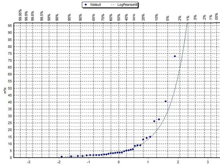
شکل ۸. برازش مقادیر حداکثر دبی سالانه با توزیع لوگ پیرسون تیب ۳ در ایستگاه گرمادشت
