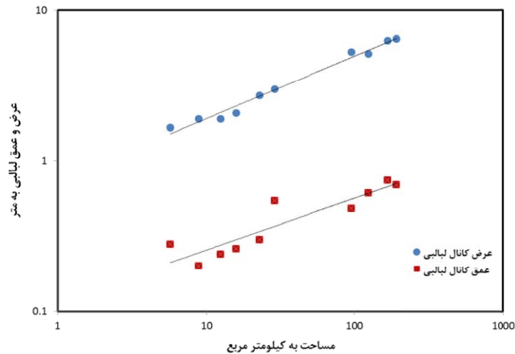
شکل ۴. نمودار لگاریتمی مساحت حوضه در مقابل عرض و عمق لبالبی حوضه گرمابدشت
