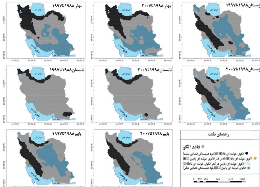
شکل ۲. نتایج به دست آمده از پراکنش الگوی موران محلی برای بارش طی دو دوره مورد مطالعه
