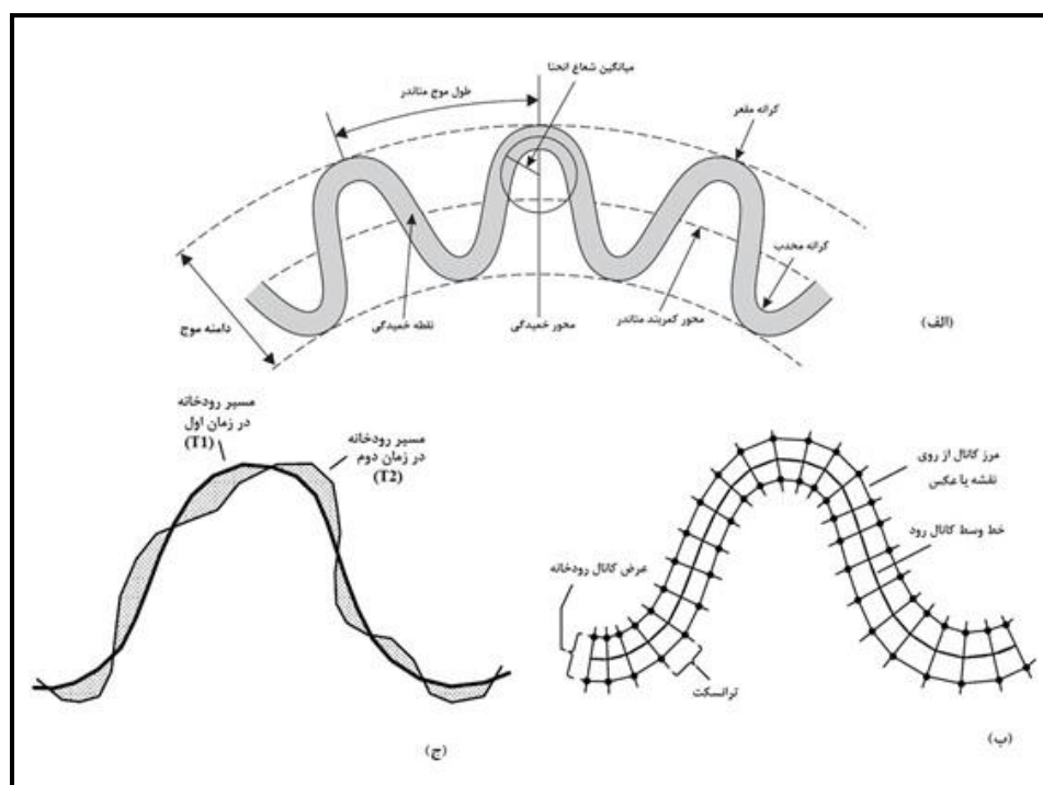
شکل ۲. روش‌های اندازه‌گیری: الف) پارامترهای هندسی پلان‌فرم رود (حسین‌زاده و اسماعیلی، ۱۳۹۴: ۲۴۳)؛ ب) عرض کانال لبابی رود؛ ج) میزان فعالیت کانال رود (مگدانلو و فرناندز، ۲۰۱۱: ۲۰۰)
