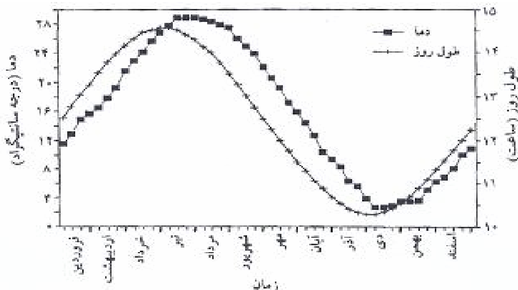
شکل ۳. روند تغییرات میانگین دما و طول روز (در محدوده شدت نور ۰/۰۰۱ کالری بر سانتی‌متر مربع بر دقیقه) طی سال در اصفهان (خواجه‌پور، ۱۳۷۷، ۳۷)
