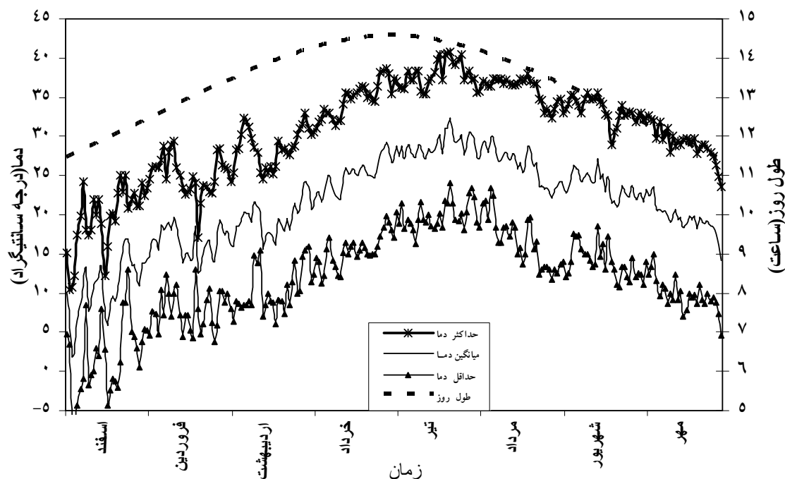
شکل ۲. روند تغییرات طول روز و دمای حداقل، حداکثر و میانگین طی فصل رشد در سال زراعی ۱۳۸۶-۸۷
