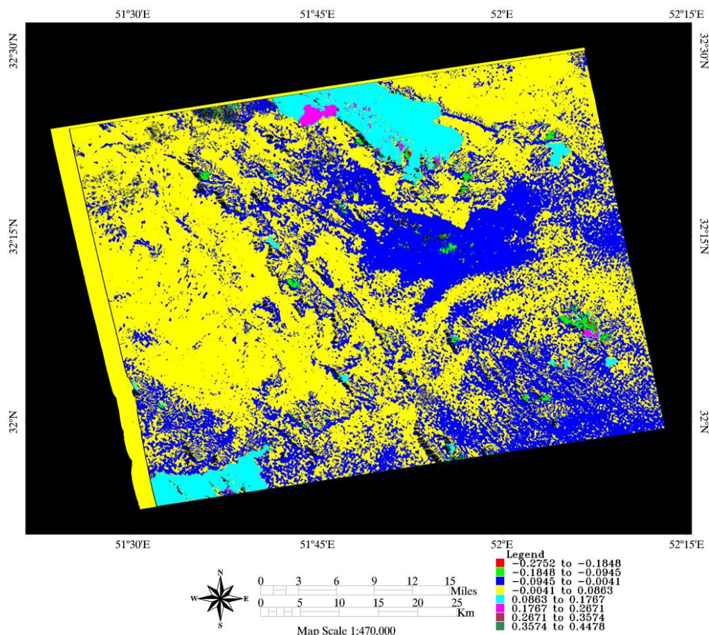
شکل ۲. نقشه‌ی میزان فرونشست و بالآمدگی دشت مهبیار (۲۰۰۹-۲۰۰۸)
