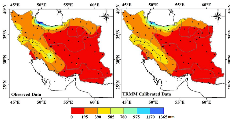
شکل ۱۰. مقایسه توزیع مکانی میانگین سالانه بارندگی در دوره ۱۹۹۸-۲۰۰۹ بر اساس مقادیر مشاهداتی (سمت چپ) و مقادیر تصحیح شده TRMM (سمت راست) در زون‌های اقلیمی ایران بر اساس روش زمین آماری کوکریجینگ
