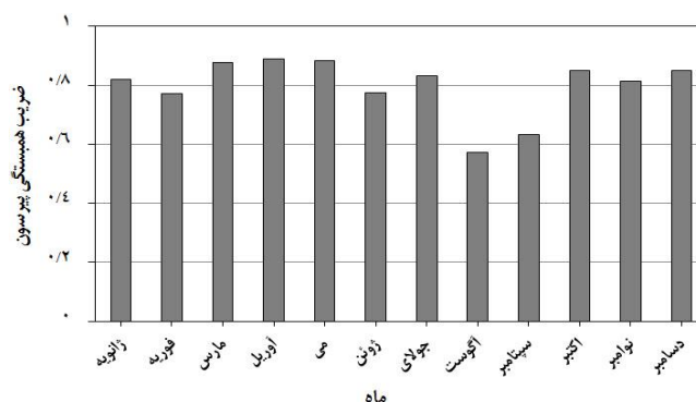
شکل ۶. همبستگی ضرایب همبستگی بین میانگین ماهانه بارندگی TRMM و مشاهده‌ای (ایران)
