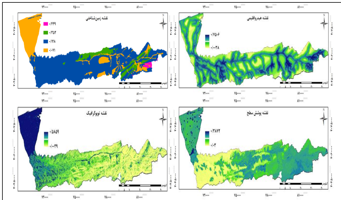
شکل ۷. نقشه‌های عوامل مؤثر در خطر سیل: هیدرواقليم، توپوگرافیک، زمین‌شناختی، و پوشش سطح
