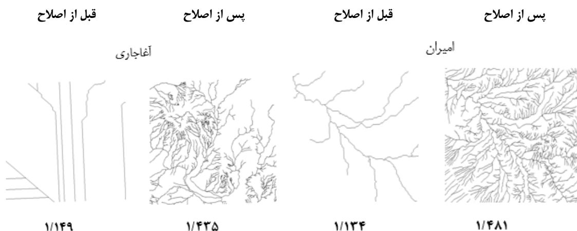
شکل ۳. بُعد فراکتال نمونه‌ای از شبکه هیدروگرافی سازند آغاچاری و امیران قبل و پس از اصلاح شبکه هیدروگرافی
