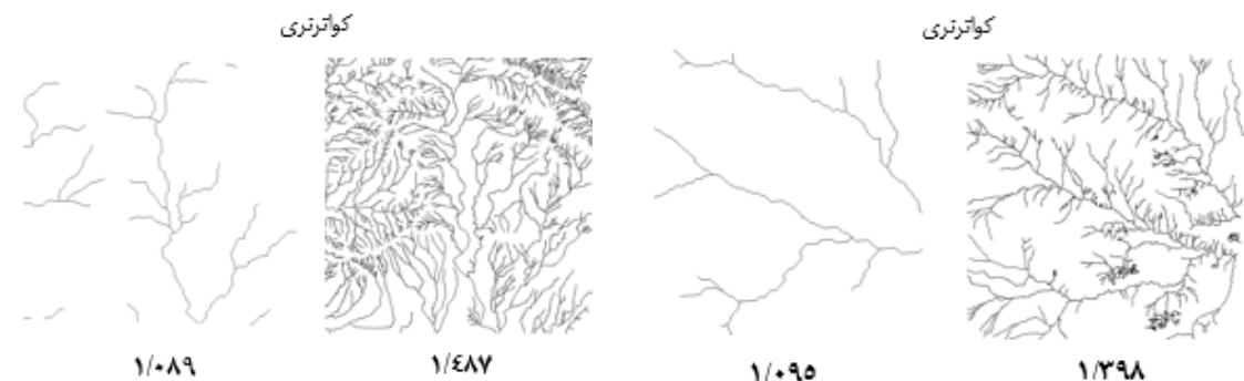
شکل ۵. بُعد فراکتال نمونه‌ای از شبکه هیدروگرافی سازند کواترنری قبل و پس از اصلاح شبکه هیدروگرافی
