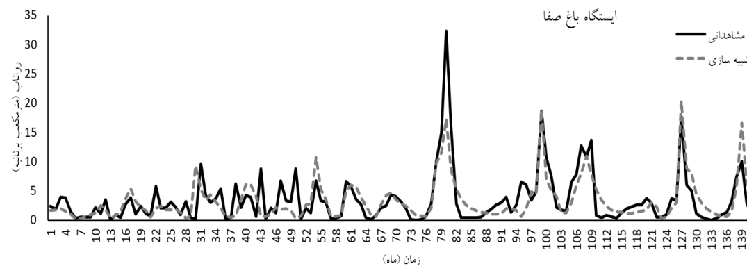
شکل ۴. سری زمانی شبیه‌سازی شده برای داده‌های مشاهده‌ای بارش
