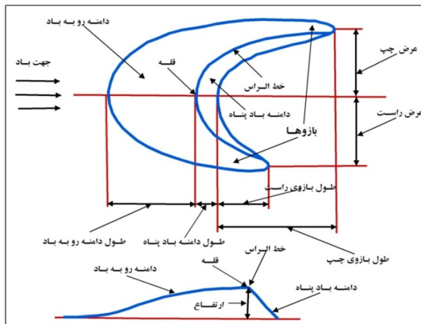
شکل ۳. توضیح تصویری مؤلفه‌های مورفومتری برخان (اقتباس از Hughe & Daniell, 2007, 642; Sauer mann et al., 2000, 48; Hesp & Hastings, 1998, 195).
