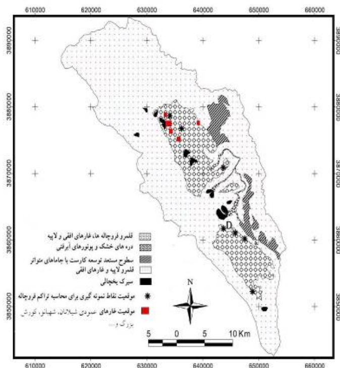
شکل ۲. نقشه ساده‌شده ژئومورفولوژی منطقه
