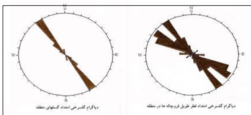
شکل ۵. نمودار گلسرخی قطر طویل فروچاله‌ها و جهت غالب گسل‌های منطقه (اقتباس از قربانی، ۱۳۸۲)
