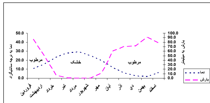
شکل ۸. نمودار آمپروترمیک منطقه (۱۳۸۶-۱۳۷۲)
