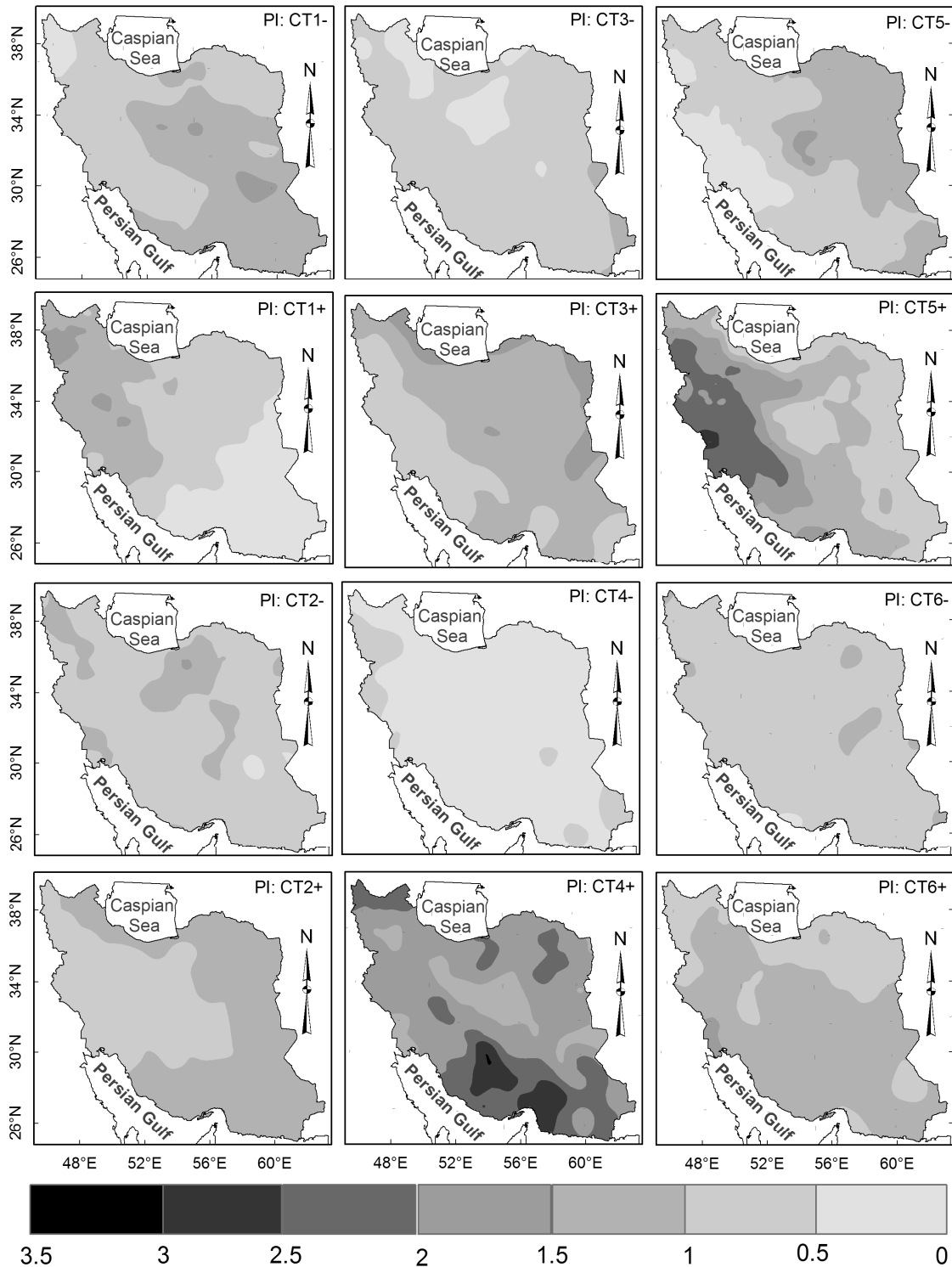
شکل ۵. توزیع ماهانه گروه‌های اصلی الگوهای گردش جوئی تراز ۵۰۰ هکتوپاسکال
