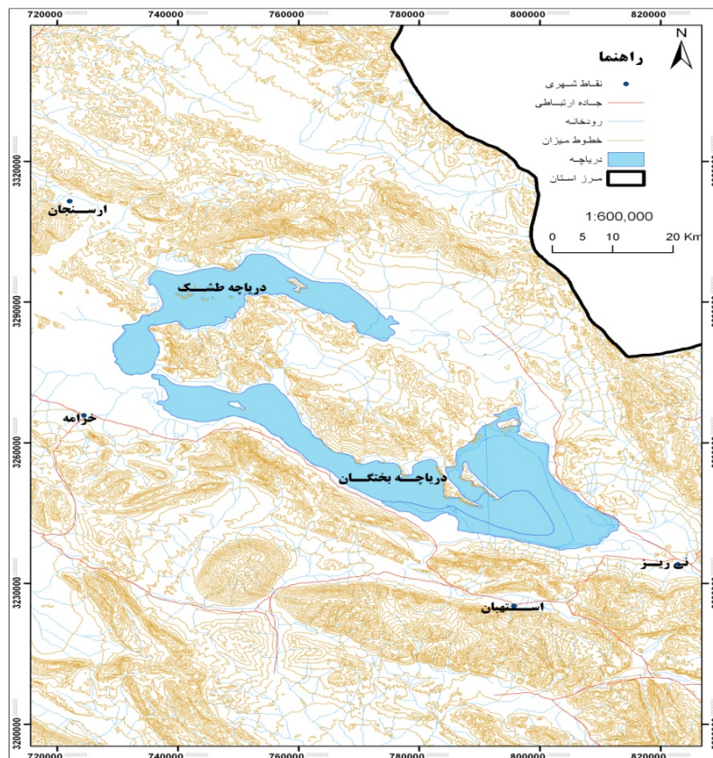
شکل ۲. وضعیت توپوگرافی دریاچه‌های طشک و بختگان
