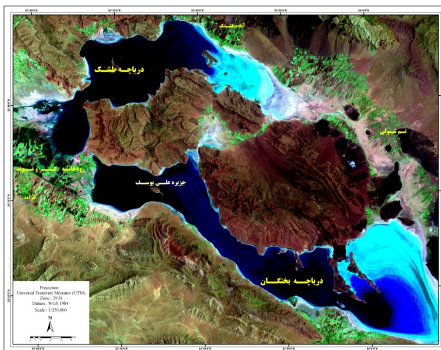
شکل ۳. تصویر ماهواره ETM از دریاچه‌های طشک و بختگان (ترکیب باندهای ۲-۵-۷)
