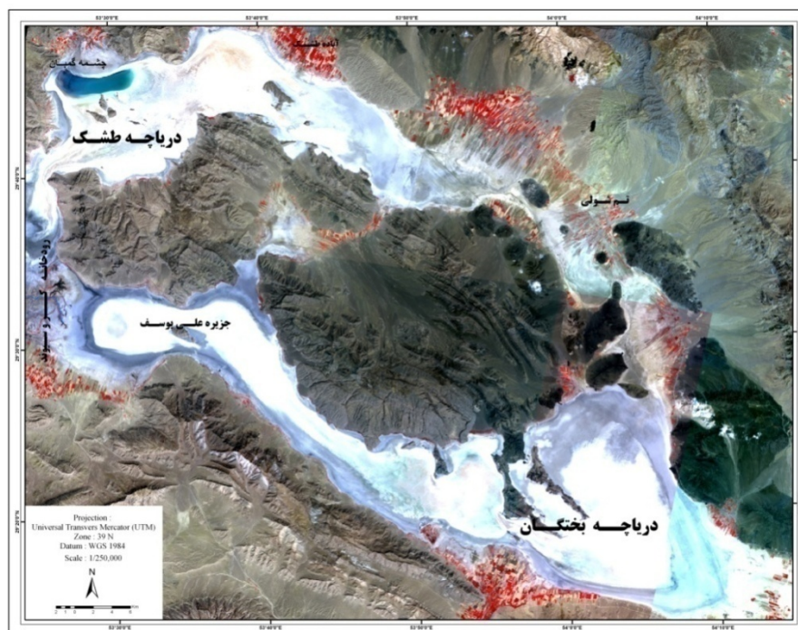
شکل ۴. تصویر ماهواره Aster از دریاچه‌های طشک و بختگان در مرداد ماه ۲۰۰۵ (ترکیب باندهای ۲-۳-۴)
