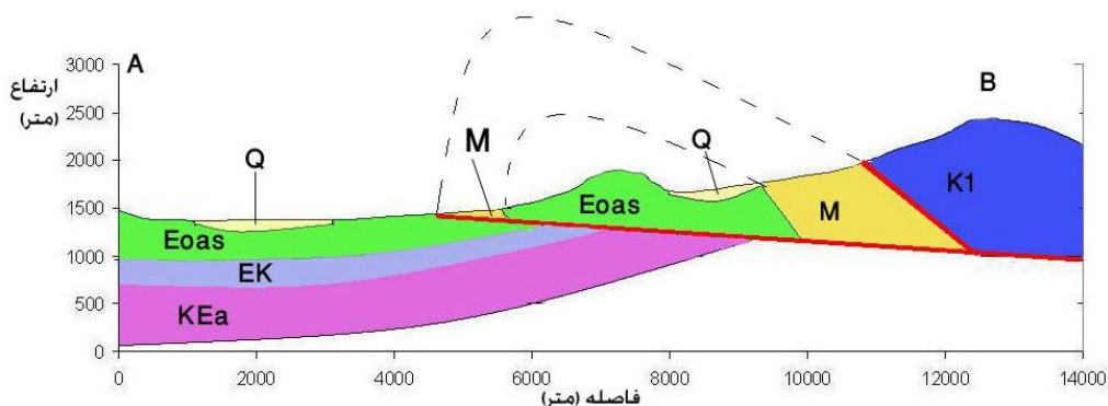
شکل ۳. مقطع زمین‌شناسی حوضه‌ی مورد مطالعه
