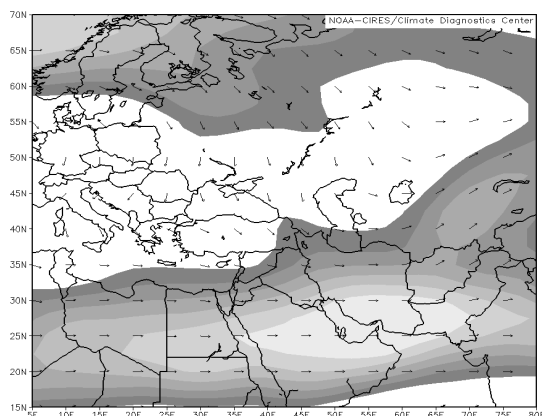
شکل ۲۲ بردار باد تراز ۵۰۰ در الگوی پرفشار آزارات.
