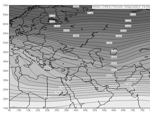
شکل ۱۶ نقشه تراز ۵۰۰ هکتوپاسکال در الگوی مداری
