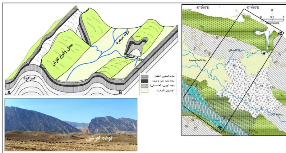
شکل ۵. بلوک دیاگرام دره‌ی رود سیمره پیش از وقوع لغزش بزرگ سیمره و نقشه‌ی زمین‌شناسی موقعیت لغزش
