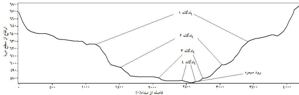
شکل ۹. نیم‌رخ عرضی سطوح پادگانه‌های دریاچه‌ای
