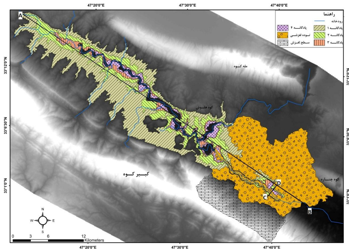
شکل ۱۳. سطوح پادگانه‌های دریاچه‌ای در منطقه‌ی مطالعاتی
