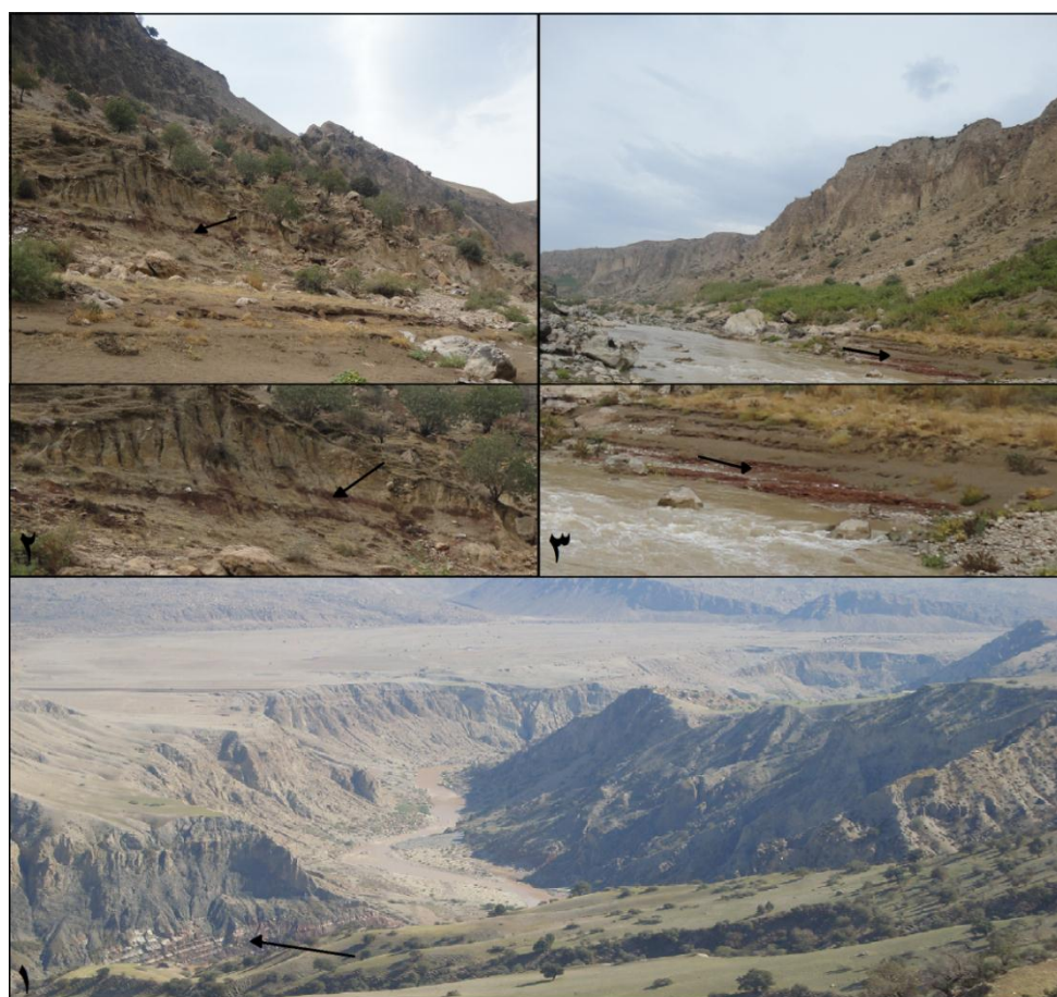
شکل ۶. سازند رسوبی قرمز رنگ سازند گچساران (توالی گچ و مارن قرمز) در زیربنای توده‌ی لغزشی قرار گرفته است. ارتفاع این لایه ۴۹۱ متر است. قسمت پایین نیز دره‌ی ایجاد شده در توده‌ی لغزشی سیمره و رسوبات لغزشی را نشان می‌دهد.
