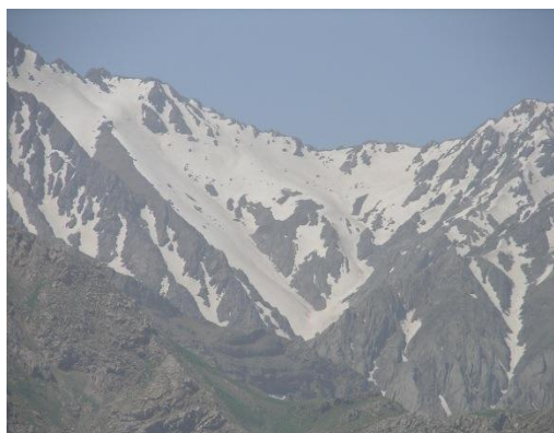
شکل ۱۰. سیرک زفره در شمال شرق کوه مارشینان
