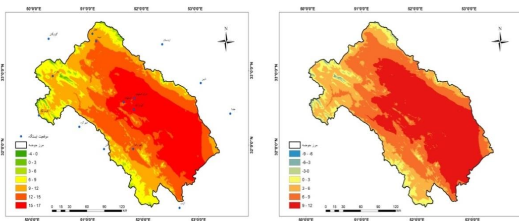
شکل ۴. نقشه هم‌دمای فعلی حوضه دریاچه گاوخونی شکل ۵. نقشه هم‌دما حوضه دریاچه گاوخونی در دوره کواترنری
