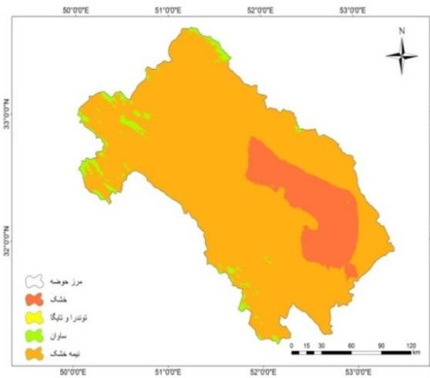
شکل ۱۴. مناطق مورفوکلیماتیکی حوضه در دوره کواترنر / شکل ۱۵. مناطق مورفوکلیماتیکی حوضه در حال حاضر
