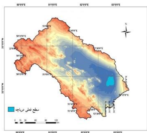
شکل ۱۷. بالاترین سطح تجربه شده دریاچه گاوخونی
