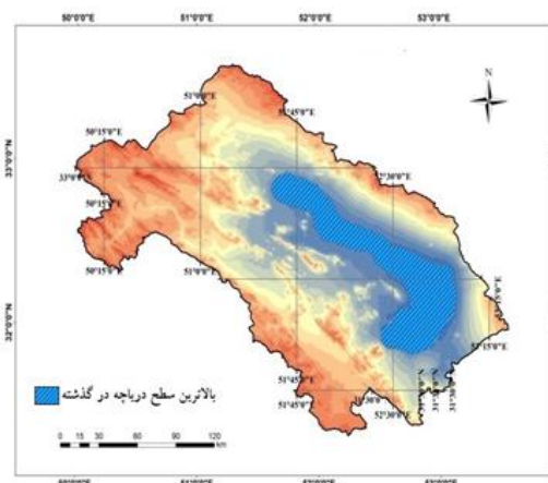
شکل ۱۸. سطح فعلی دریاچه گاوخونی
