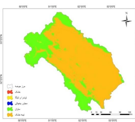
شکل ۱۴. مناطق مورفوکلیماتیکی حوضه در دوره کواترنر / شکل ۱۵. مناطق مورفوکلیماتیکی حوضه در حال حاضر
