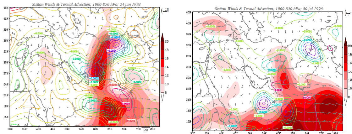
شکل ۱. بردارهای سرعت و جهت باد (m/s) و هسته‌های بیشینه سرعت باد (هاشورهای رنگی) تراز ۸۵۰ ه.پ؛ مجموع وزش دمایی (10^{-5} s^{-1}) * C^{\circ} ترازهای ۹۲۵-۱۰۰۰ و ۸۵۰-۹۲۵ ه.پ؛ الف) الگوی همید ۱، ۲۴ ژوئن ۱۹۹۳؛ ب) الگوی همید ۲، ۳۰ ژوئیه ۱۹۹۶
