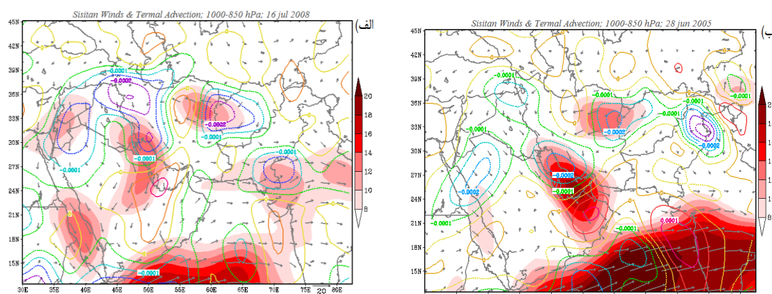
شکل ۲. بردارهای سرعت و جهت باد (m/s) و هسته‌های بیشینه سرعت باد (هاشورهای رنگی) تراز ۵۸۵۰ ه.پ؛ مجموع وزش دمایی (10^{-5} \text{ s}^{-1}) \times \text{C}^{\circ} ترازهای ۹۲۵-۱۰۰۰ و ۸۵۰-۹۲۵ ه.پ؛ الف) الگوی همدید ۳، ۱۶ ژوئای ۲۰۰۸؛ ب) الگوی همدید ۴، ۲۸ ژوئن ۲۰۰۵
