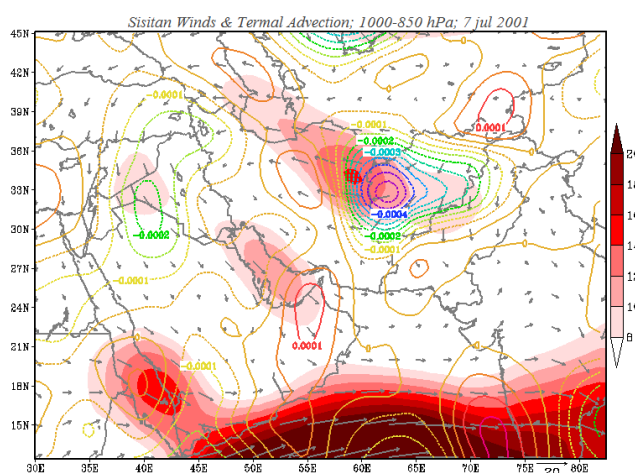
شکل ۳. بردارهای سرعت و جهت باد (m/s) و هسته‌های بیشینه سرعت باد (هاشورهای رنگی) تراز ۵۸۵۰ ه.پ؛ مجموع وزش دمایی (10^{-5} \text{ s}^{-1}) \times \text{C}^{\circ} ترازهای ۹۲۵-۱۰۰۰ و ۸۵۰-۹۲۵ ه.پ؛ الگوی همدید ۵، ۷ ژوئای ۲۰۰۱
