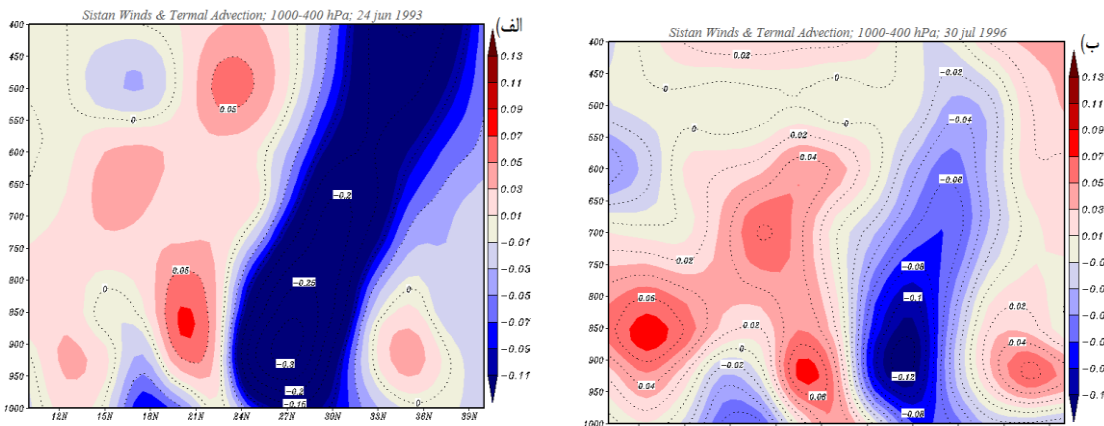
شکل ۷. نیمرخ ارتفاعی وزش دمایی جو (Co*10-5s-1) از مدار 10^{\circ}N تا 40^{\circ}N در امتداد نصف‌النهار 60^{\circ}E ، از تراز ۴۰۰-۱۰۰۰ ه.پ؛ الف) الگوی همدید ۱، ۲۴ ژوئن ۱۹۹۳؛ ب) الگوی همدید ۲، ۳۰ ژوئیه ۱۹۹۶
