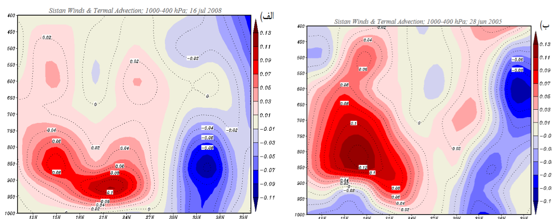
شکل ۸. نیمرخ ارتفاعی وزش دمایی جو ( Co*10-5s-1 ) از مدار 10^{\circ}N-40^{\circ}N در امتداد نصف‌النهار Eo 6^{\circ} ، از تراز 400-1000 ه.پ؛ الف) الگوی همیدید ۳، ۱۶ ژوئیه ۲۰۰۸؛ ب) الگوی همیدید ۴، ۲۸ ژوئن ۲۰۰۵
