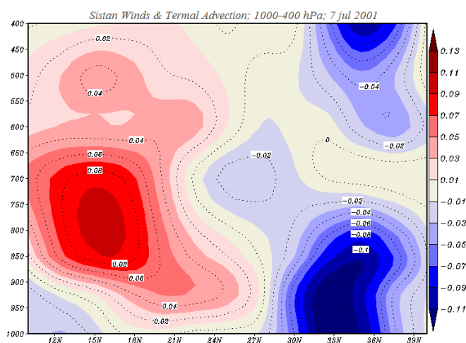
شکل ۹. نیمرخ ارتفاعی وزش دمایی جو ( Co*10-5s-1 )، از مدار 10^{\circ}N-40^{\circ}N در امتداد نصف‌النهار Eo 6^{\circ} ، از تراز 400-1000 ه.پ؛ الگوی همیدید ۵، ۷ ژوئیه ۲۰۰۱
