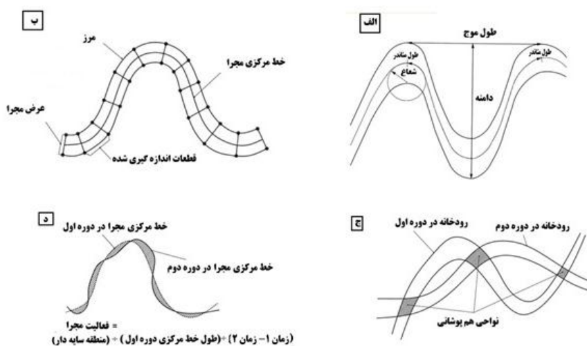
شکل ۳. نمایش شماتیک از اجزای اندازه‌گیری شده مائند رودخانه (تسیلد و همکاران، ۲۰۰۰؛ ریچارد و همکاران، ۲۰۰۵)
