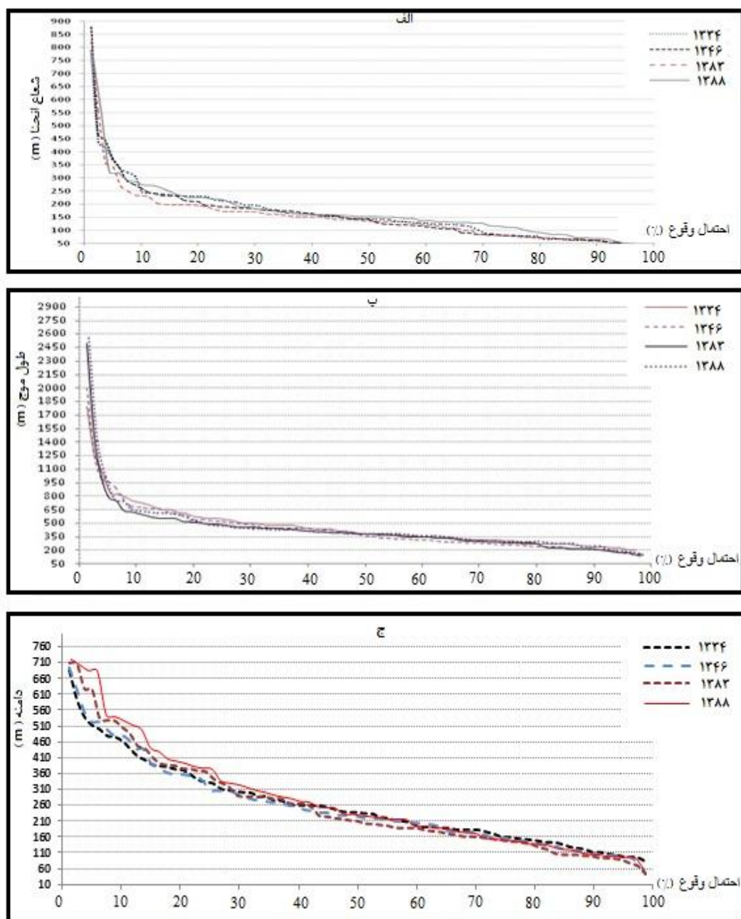
شکل ۶. نمودار درصد احتمال رخداد شعاع انحنای موج، و دامنه قوس رودخانه قره‌سو در چهار دوره زمانی
