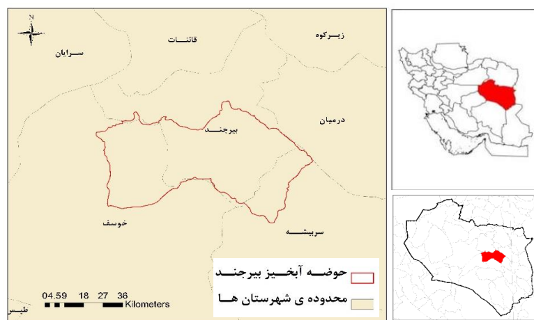
شکل ۱. نقشه موقعیت حوضه آبخیز بیرجند
