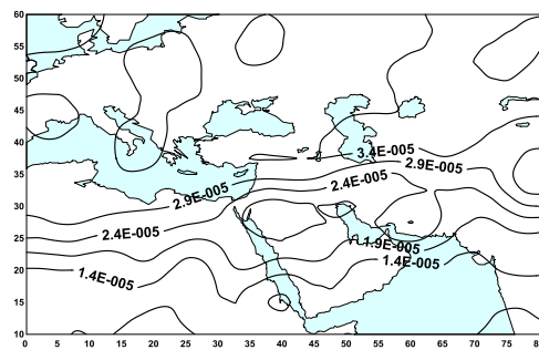
شکل ۹. توزیع مکانی تاوایی پتانسیلی راسبی- ارتل تراز ۵۰ هکتوپاسکال در ساعت ۰۰۰۰ گرینویچ روز ۱۹۷۴/۱۲/۵
