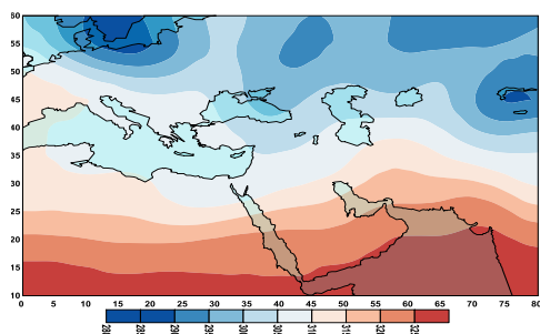
شکل ۱۲. الگوی دمای پتانسیل تراز ۵۰ هکتوپاسکال بر حسب کلون ساعت ۱۲۰۰ گریجوی ۱۹۷۴/۱۲/۵
