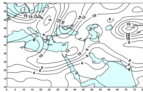
شکل ۷. توزیع مکانی تاوایی مطلق تراز ۵۰۰ هکتوپاسکال بر حسب 10^{-5} s^{-1} در ساعت ۰۰۰۰ گرینویچ روز ۱۹۷۴/۱۲/۵
