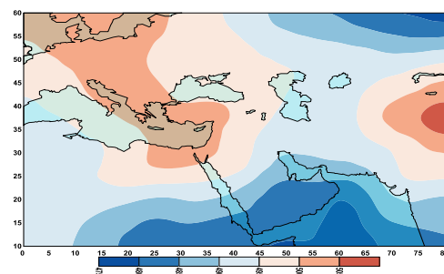
شکل ۱۱. الگوی دمای پتانسیل تراز ۵۰ هکتوپاسکال بر حسب کلون در ساعت ۱۲۰۰ گریجوی ۱۹۷۴/۱۲/۵
