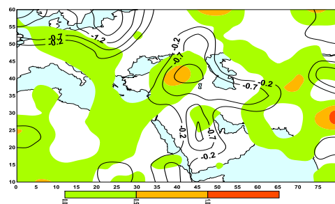
شکل ۱۳. همگرایی تراز ۱۰۰۰ هکتوپاسکال (پهنه‌های رنگی) و واگرایی تراز ۵۰۰ هکتوپاسکال (خطوط هم‌مقدار) بر حسب 10^{-10} \text{ s}^{-1} ساعت ۱۲۰۰ گرینویچ روز ۱۹۷۴/۱۲/۵
