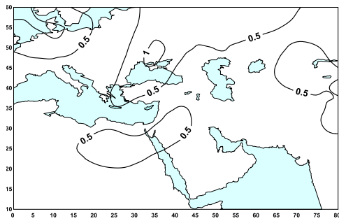
شکل ۸. توزیع مکانی تاوایی پتانسیلی راسبی- ارتل تراز ۵۰۰ هکتوپاسکال بر حسب 10^{-5} s^{-1} در ساعت ۰۰۰۰ گرینویچ روز ۱۹۷۴/۱۲/۵
