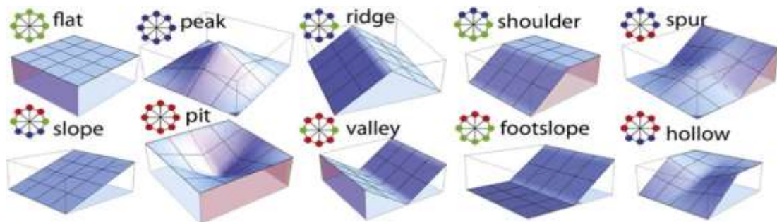
شکل ۴. ده ژئومورفون غالب در چشم‌انداز (جاسویز، ۲۰۱۳)
