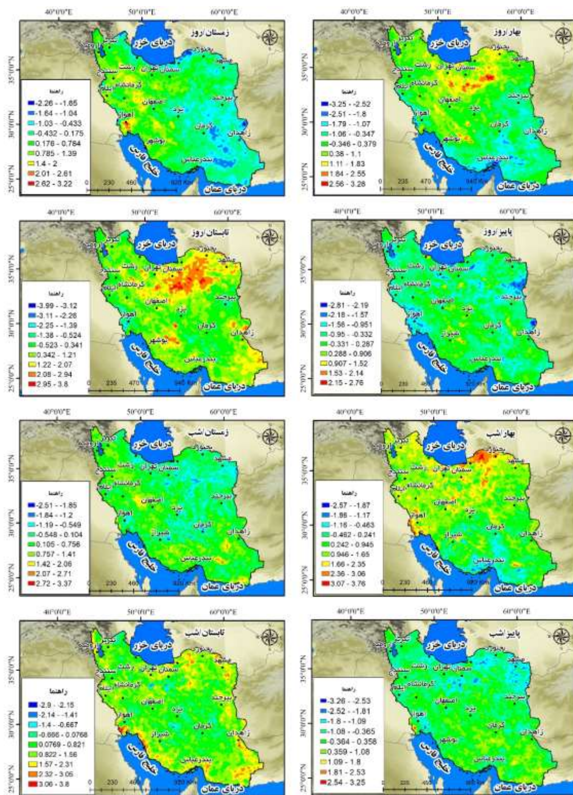
شکل ۲. بی‌هنجاری فصلی بلندمدت (۲۰۰۱-۲۰۱۸) در روز و شب با استفاده از داده‌های سنجنده MODIS (واحد اعداد راهنما: درجه سلسیوس)
