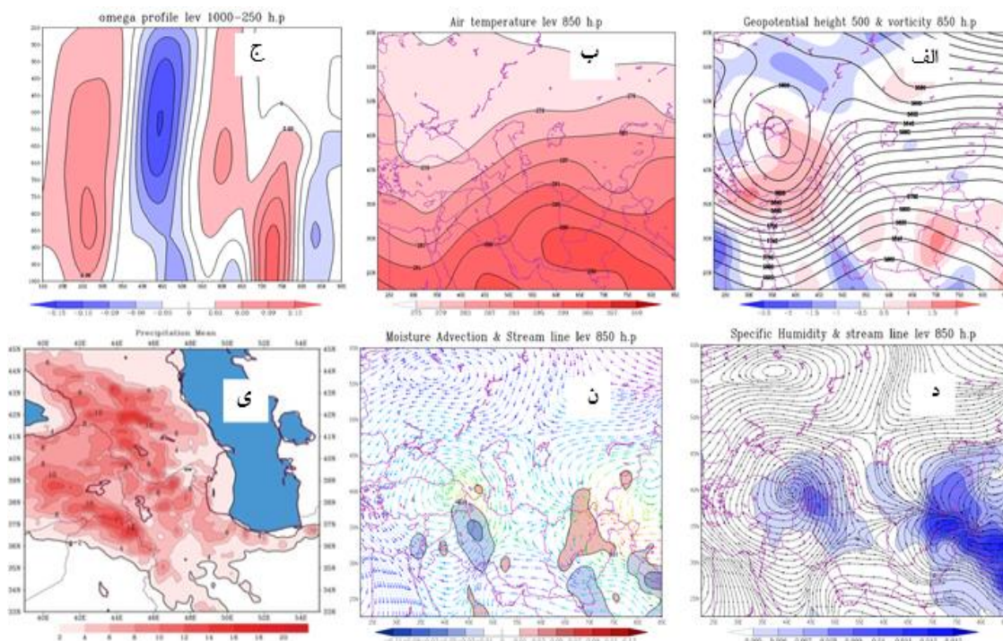
شکل شماره ۷. الگوی هم‌مدید بندالی: الف) نقشه ترکیبی ارتفاع ژئوپتانسیل تراز ۵۰۰ ه.پ و تاوایی نسبی تراز ۸۵۰ ه.پ؛ ب) دمای هوای تراز ۸۵۰ ه.پ؛ ج) نیمرخ مؤلفه امگا یا جریان قائم هوا در تراز ۱۰۰۰ تا ۲۵۰ ه.پ؛ د) رطوبت ویژه و خطوط جریان تراز ۸۵۰ ه.پ؛ ن) وزش رطوبت تراز ۸۵۰ ه.پ؛ ی) میانگین بارش
