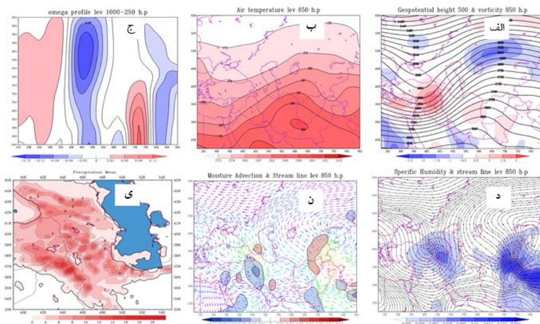
شکل شماره ۸. الگوی ناوه شرقی مدیترانه: الف) نقشه ترکیبی ارتفاع ژئوپتانسیل تراز ۵۰۰ ه.پ و تاوایی نسبی تراز ۸۵۰ ه.پ؛ ب) دمای هوا تراز ۸۵۰ ه.پ؛ ج) نیمرخ مؤلفه امگا یا جریان قائم هوا در تراز ۱۰۰۰ تا ۲۵۰ ه.پ؛ د) رطوبت ویژه و خطوط جریان تراز ۸۵۰ ه.پ؛ ن) وزش رطوبت تراز ۸۵۰ ه.پ؛ ی) میانگین بارش
