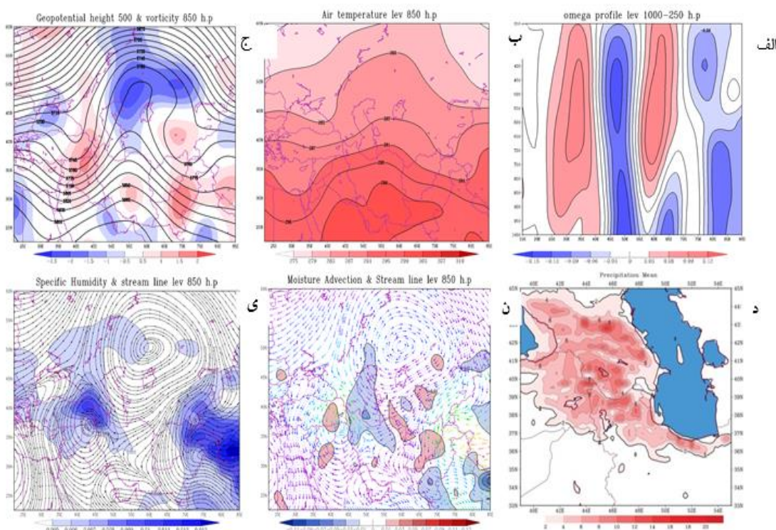
شکل ۴. الگو ناوهٔ عمیق: الف) نقشهٔ ترکیبی ارتفاع ژئوپتانسیل تراز ۵۰۰ ه.پ و تاوایی نسبی تراز ۸۵۰ ه.پ؛ ب) دمای هوا تراز ۸۵۰ ه.پ؛ ج) نیمرخ مؤلفهٔ امگا یا جریان قائم هوا در تراز ۱۰۰۰ تا ۲۵۰ ه.پ؛ د) رطوبت ویژه و خطوط جریان تراز ۸۵۰ ه.پ؛ ن) وزش رطوبت تراز ۸۵۰ ه.پ؛ ی) میانگین بارش
