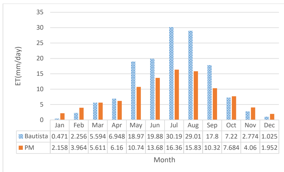
شکل ۸. میانگین تبخیر-تعرق ماهانه فائو پن من مانتت و باتیستا و همکاران (۲۰۰۹)
