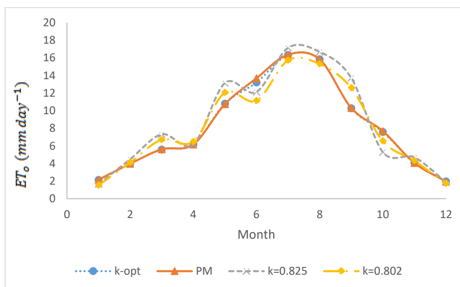
شکل ۱۰. مقدار تبخیر-تعرق به دست آمده با روش ترون‌ت‌وایت بر اساس مقادیر مختلف ضریب k در ماه‌های مختلف سال در مقایسه با روش فائو پن-من-مانتث
