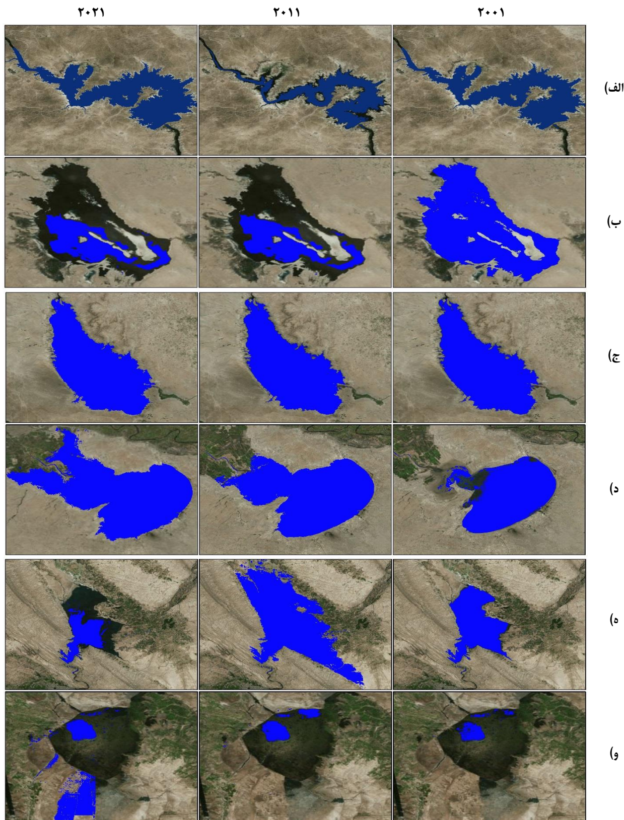
شکل ۲. تغییرات زمانی-فضایی بدنه‌های آبی دجله و فرات (الف: دریاچه قادسیه، ب: دریاچه رزازه، ج: دریاچه ثرثار، د: دریاچه حبانیه، ه: دریاچه حمین، و: تالاب هورالعظیم)
